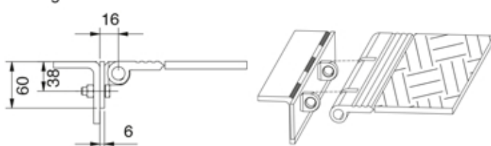
Ausführung 3 Durchgehendes Stahlteil zum Anschweißen/Anschrauben
