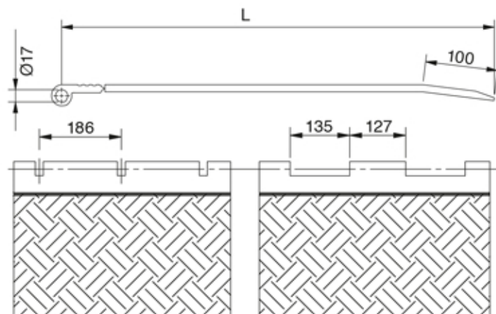
Ausführung 1 Aluminium Profilabschnitte zum Anschrauben
