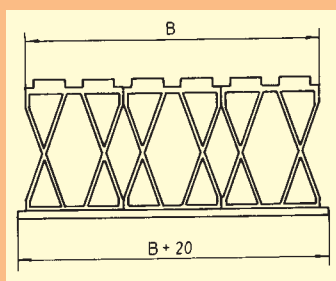
Příčný řez profilem VRV 185
